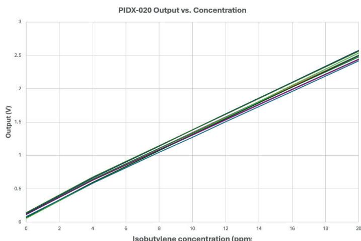
Fig. 1 PIDX-A-020线性度 (0-20 ppm)
